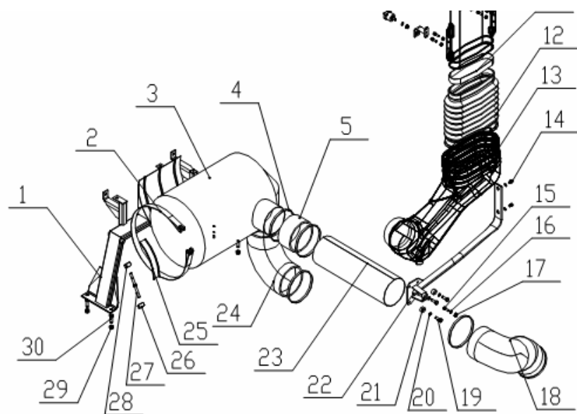
HW 空滤器FDJF06
