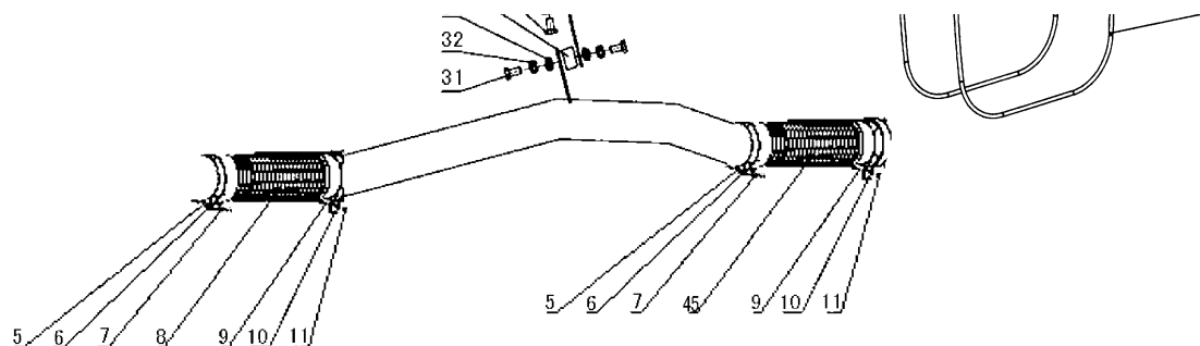
HW 排气管及消声器FDJF05
