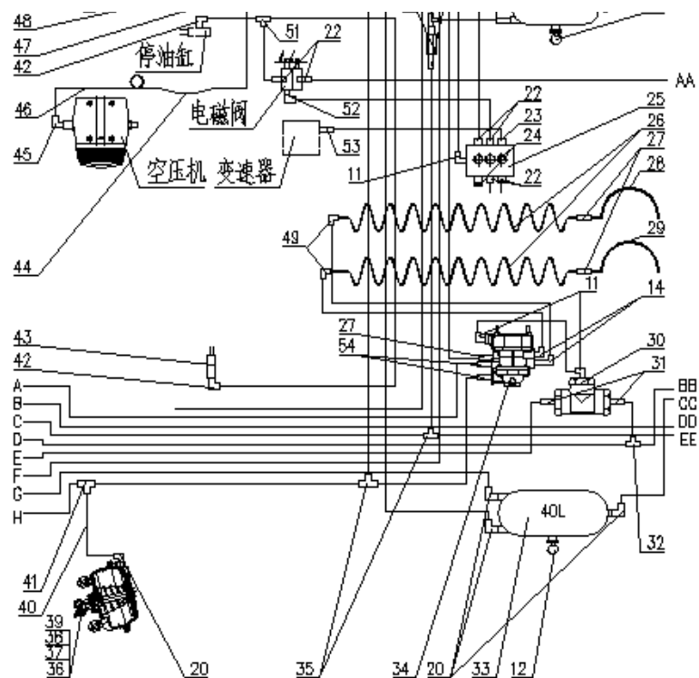
HW 底盘前部制动ZD02
