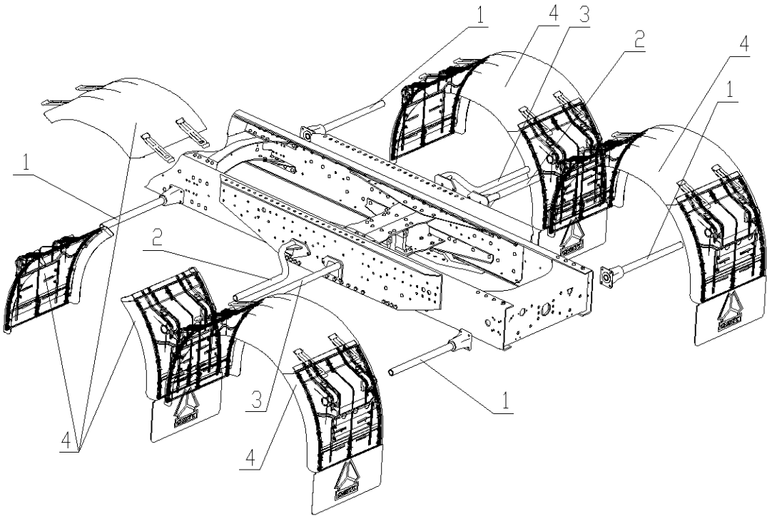
牵引车后挡泥板XG04B
