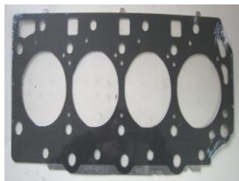
汽缸盖垫：1片/台 材质：金属
