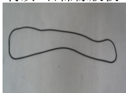
时规橡皮: 1条/台 材质: NBR
