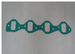
进气支管垫: 1片/台 材质: 石棉橡胶板
